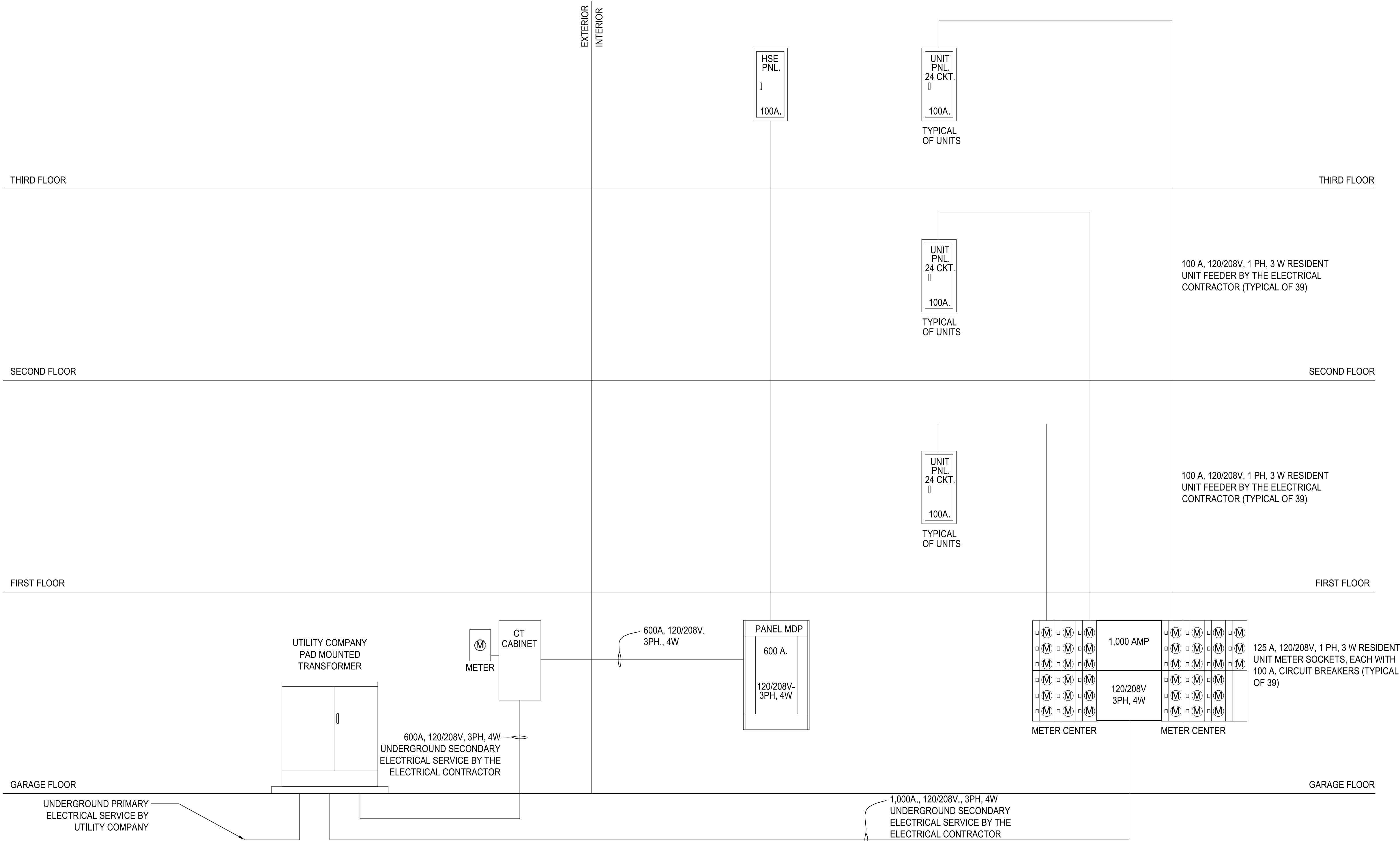
1 ELECTRICAL RISER DIAGRAM SCALE: N.T.S.
